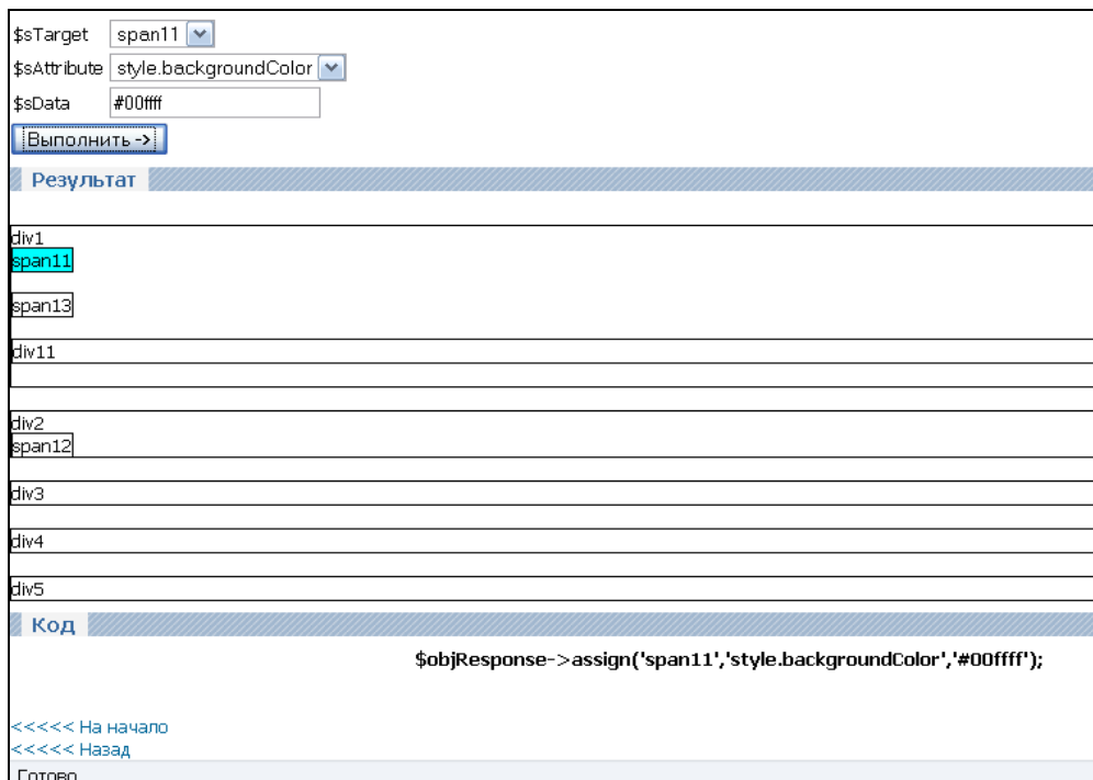
Рис. 1.5. Вид страницы после выполнения функции assign()
