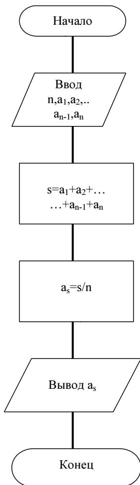
Рис. 1.2. Графическая схема нахождения среднего арифметического
