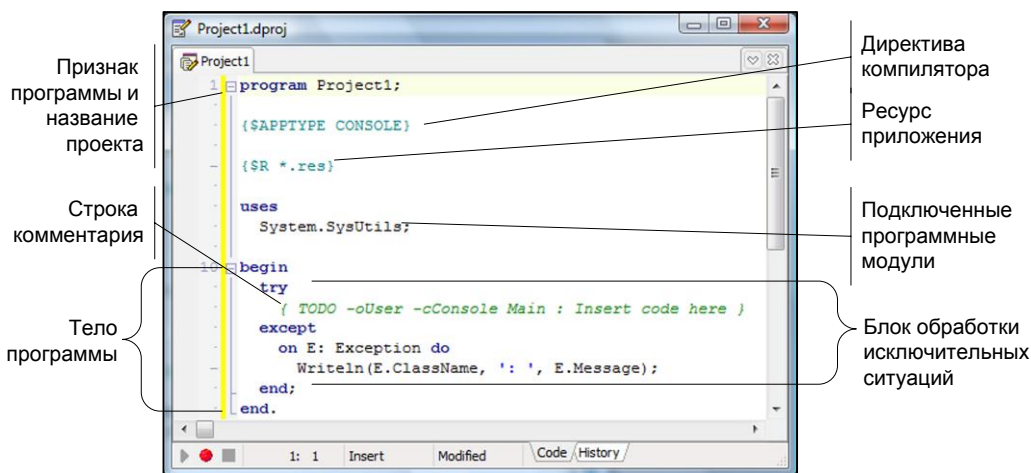
Рис. 1.2. Код консольного приложения Delphi XE2
