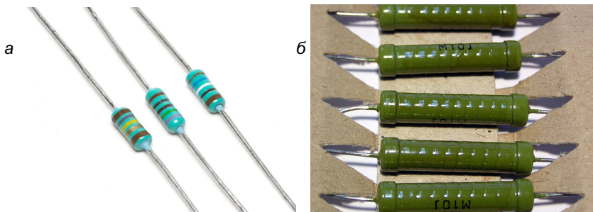
Рис. 1.3. Маркировка резистора: цветовая ( а ), буквенно-цифровая ( б )
