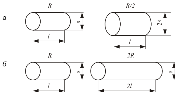
Рис. 1.1. Изменение сопротивления проводника при увеличении его площади поперечного сечения (а) и длины (б)
