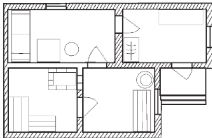
Рисунок 1. Вариант расположения комнат в небольшой бане
